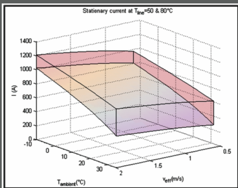
Εικόνα 1: Ρεύμα σταθερής κατάστασης που απαιτείται για τη θέρμανση του αγωγού στους 50 και 80 °C σε διαφορετικές συνθήκες περιβάλλοντος
